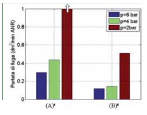
7. Portata di fuga per due diverse lamine: lamina spessa e bordo squadrato (A), lamina sottile e bordo arrotondato (B), cilindri senza asta di alesaggio 50 mm.
